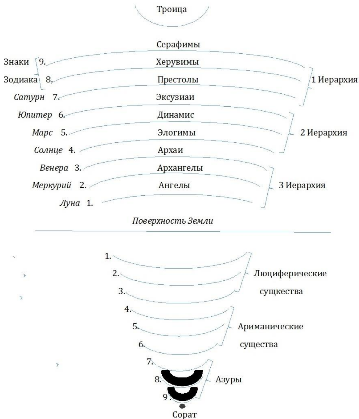
Илл. 7. Слои Земли
